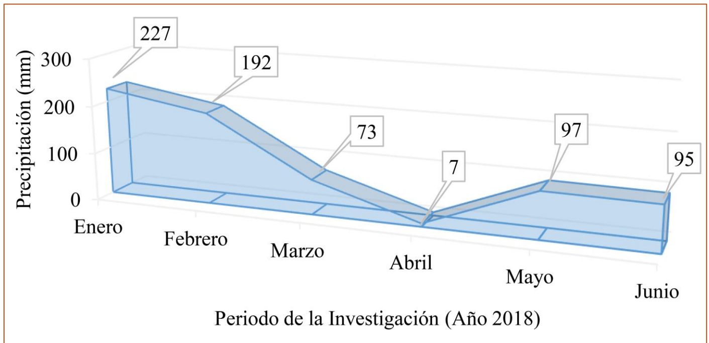
Figura 1. Datos de precipitación mensual registrada en el Distrito de Villa del Rosario, Dpto. San Pedro, durante el periodo de investigación (enero 2018 a junio 2018), proveído por la Cooperativa Volendam. Departamento de San Pedro, Paraguay, 2018.
