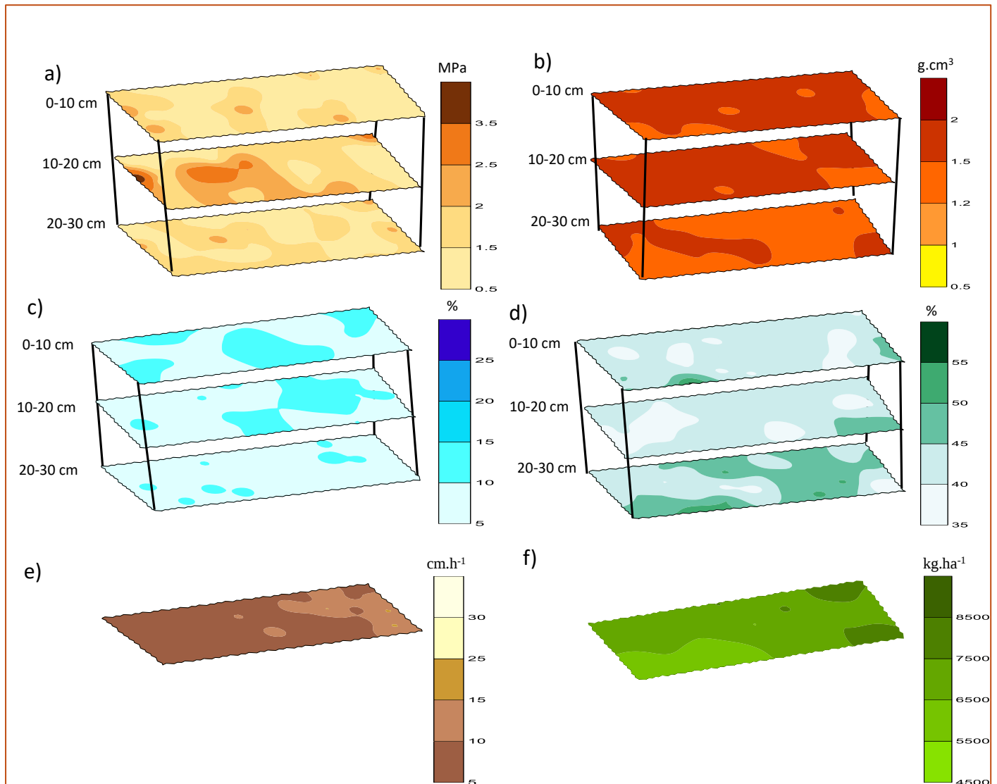
Figura 2. a) Mapa de distribución espacial de la a) resistencia mecánica a la penetración del suelo (RMPS) (MPa), b) Densidad Aparente del suelo (DAP) ( \text{g.cm}^{-3} ) c) Porosidad total del suelo (PT) (%), d) Humedad gravimétrica (Hg) (%), e) Velocidad de infiltración del agua en el suelo (VIA) ( \text{cm.h}^{-1} ), y f) Rendimiento de granos (RG) del maíz ( \text{kg.ha}^{-1} ) Departamento de San Pedro, Paraguay, 2018.
