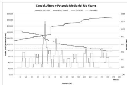
Figura 5 (b). Potencial Hidroenergético con L = 5 km
