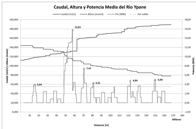
Figura 7. Potencial Hidroenergético identificado en el Río Ypané.
