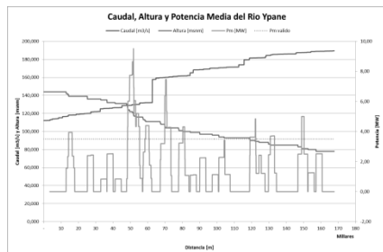
Figura 5 (a). Potencial Hidroenergético con L = 3,5 km
