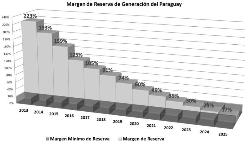
Figura 1. Margen de Generación del Paraguay
