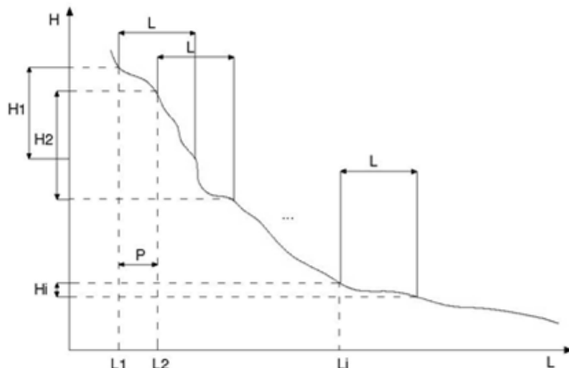
Figura 4. Curvas de Perfil Longitudinal del Río y Potencial Hidráulico
