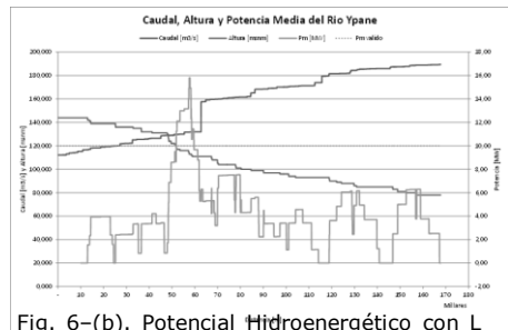
Fig. 6-(b). Potencial Hidroenergético con L = 10 km
