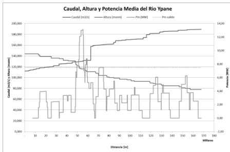
Figura 6(a). Potencial Hidroenergético con L = 7,5 km
