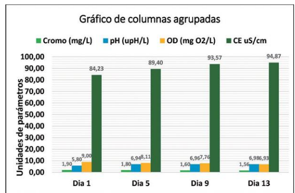
Figura 9. Variabilidad de concentración de cromo vs pH, CE y OD en los diferentes tiempos de exposición.
