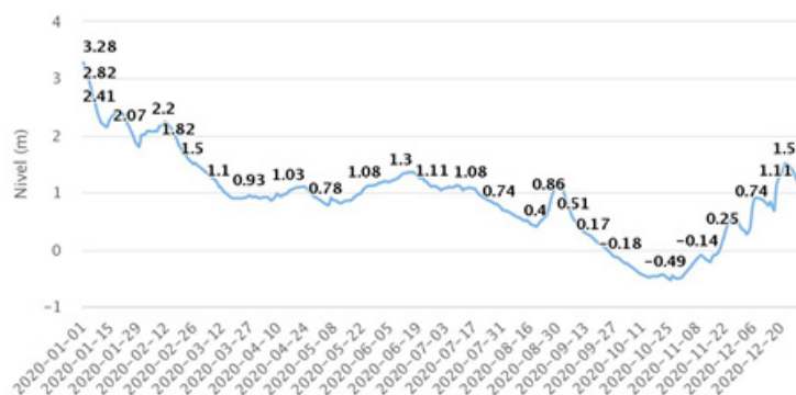
Figura 2: Nivel de altura del río en Paraguay, periodo 1-1-2020 al 31-12-2020
